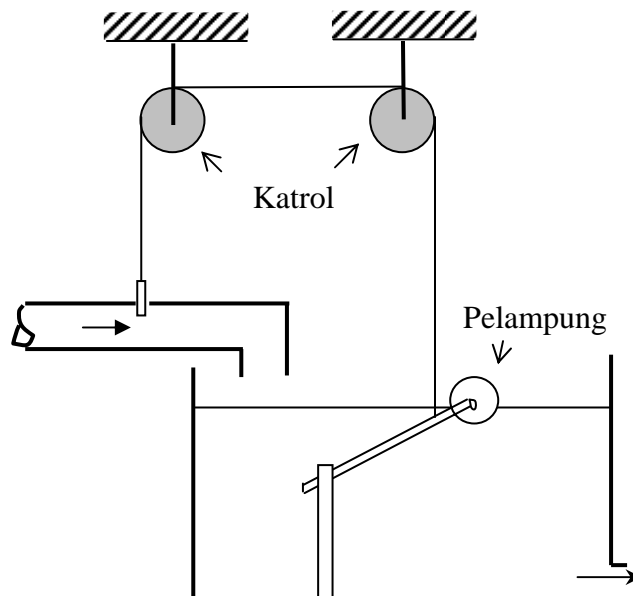
Gambar S1-1 Sistem kontrol tinggi muka
