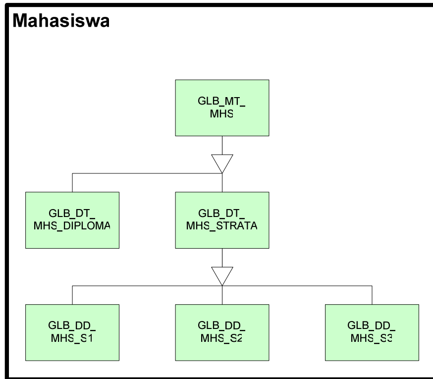
Gambar B-3.2. Diagram E-R untuk mahasiswa
