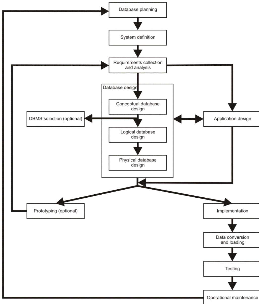
Gambar 3.2 Siklus hidup aplikasi basis data (Conolly-Begg, 2002).
